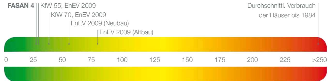
Vereinfachte Darstellung des Jahres-Primärenergieverbrauchs in kWh/(m²a)
